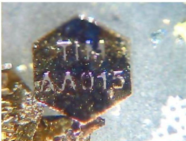
Figur 6 0,5 mm markör, lämplig för märkning av vapen och ammunition. Denna markör har bränts vid hög temperatur.
